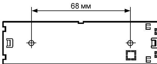
Рис.9 Присоединительные размеры
