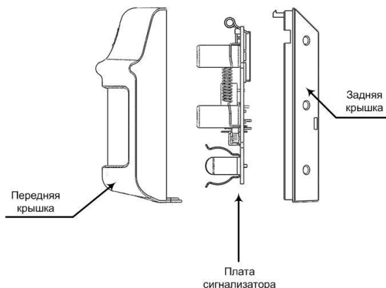
Рис.1 Конструкция сигнализатора
