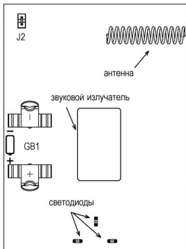
Рис. 2 Плата сирены
